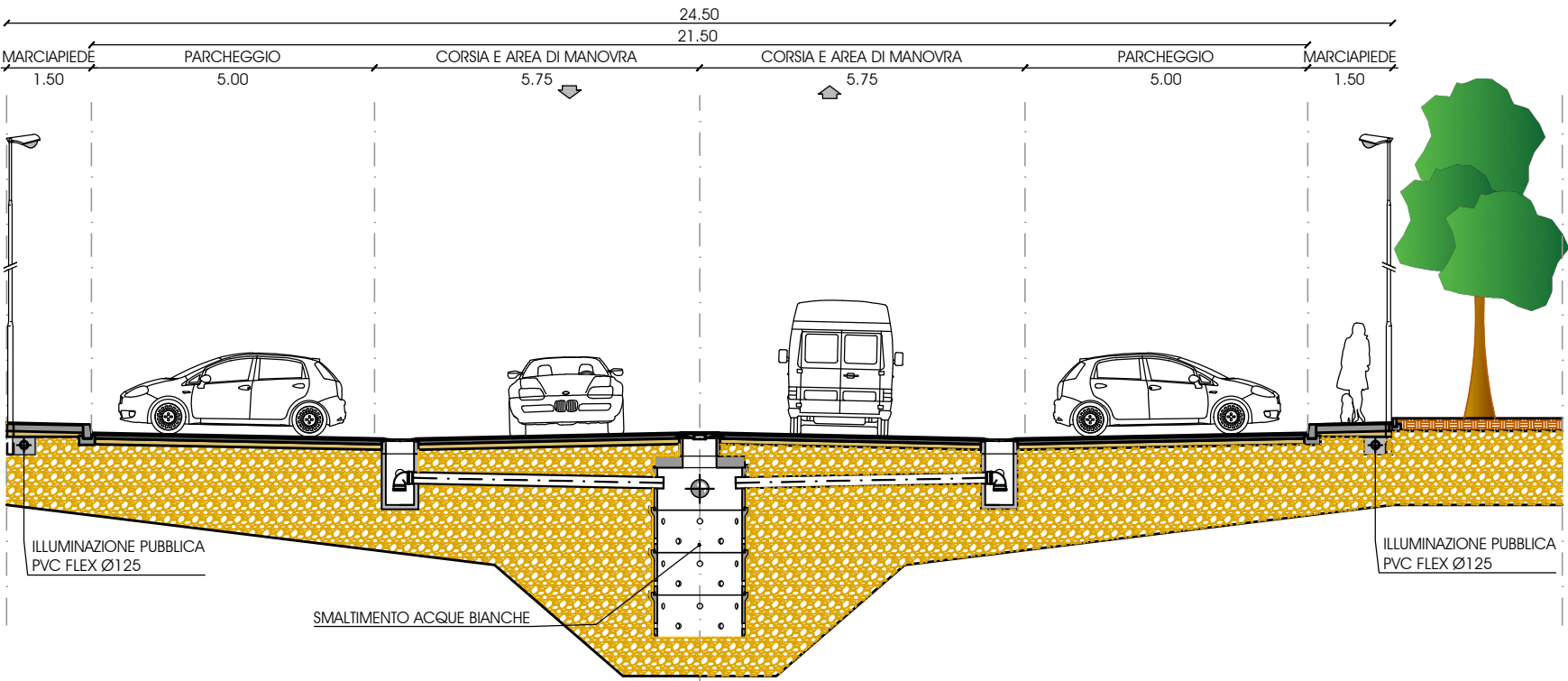
Sezione tipo parcheggio - sc. 1:100
