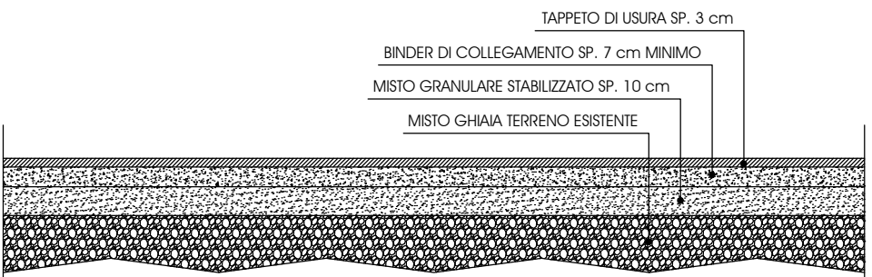
Particolare pavimentazione - sc. 1:20
